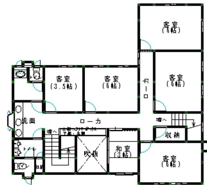
2階平面図
