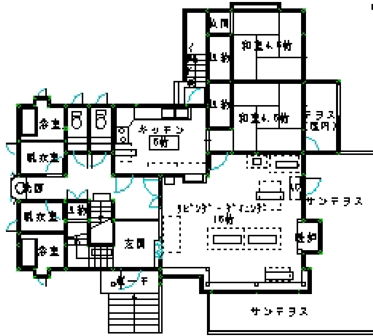
1階平面図
